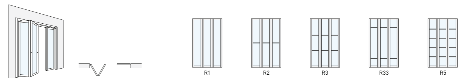
Porte a libro a tre ante (di cui una semi-fissa) / Three-wing centre split folding doors (one semi-fixed wing)
