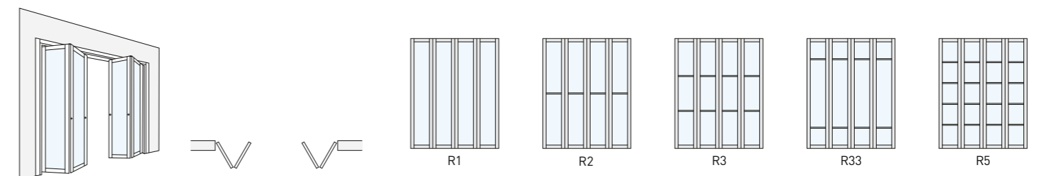
Porte a libro doppie / double folding doors
